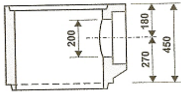
Skruž horná 5c
