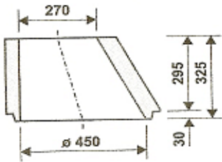
Skruž stredová 6b
