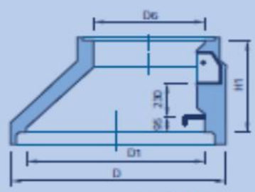
šachťový kónus
