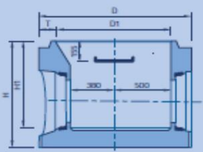
šachťová dno
