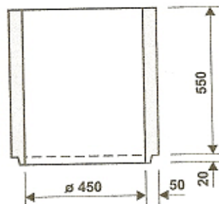
Skruž horná 5d
