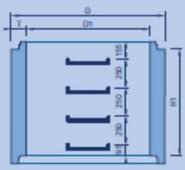
šachťová skruž
