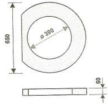
Dno s kalovou priehlbinou 2a
